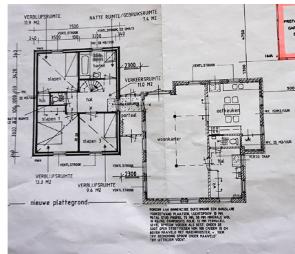
Ontwerptekening nieuwe begane grond, na verbouwing, 2000 (rechts stelp, links aanbouw uit 2000) particuliere collectie eigenaar Stoomweg 59)
