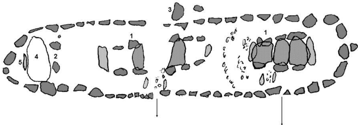
Schematisch overzicht van hunebed D43 op de Schimmeres te Emmen, met een lengte van 40,3 meter en breedte van 6,8 meter. Onderzocht in 1913 en gerestaureerd in 1960.
